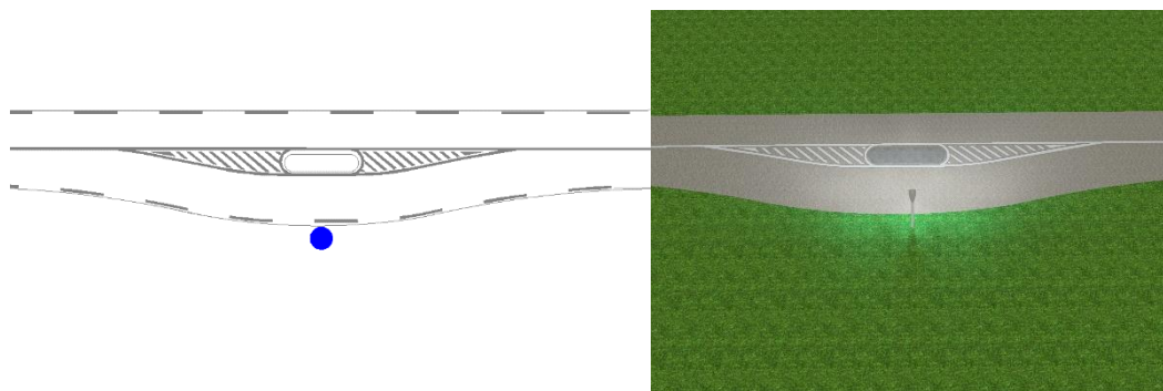
Slika 40: Primer postavitve svetilk za osvetlitev deniveliranega otoka za zamik osi smernega vozišča iz ene strani ceste
