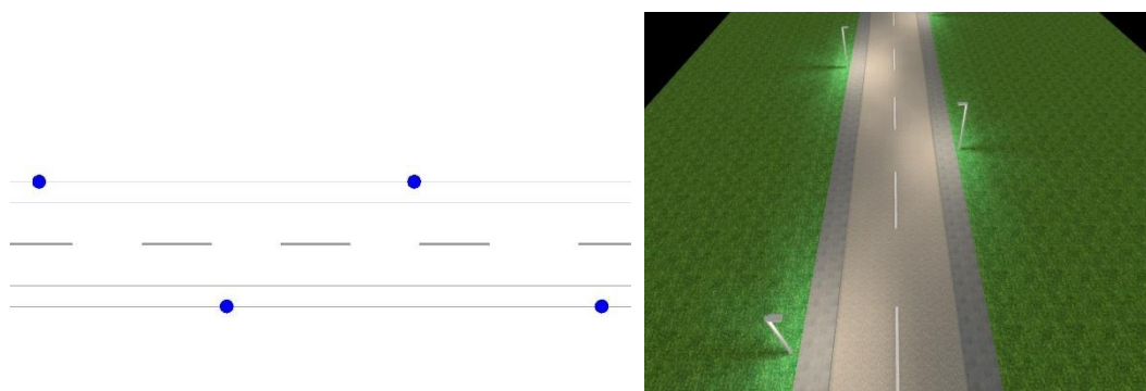
Slika 12: Primer postavitve zamaknjenih svetilk na obeh straneh ceste za osvetlitev površin za pešce na neobremenjenem delu ceste v naselju
