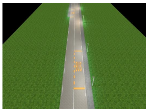
Slika 24: Primer postavitve svetilk za osvetlitev avtobusnih postajališč na neobremenjenem delu ceste v naselju z dvema svetilkama
