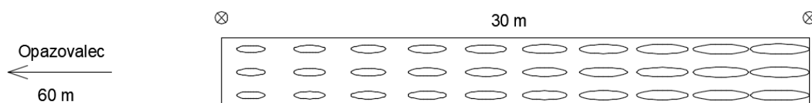
Slika 42: Velikost površine merilnih točk pri meritvi svetlosti z ustreznim inštrumentom
