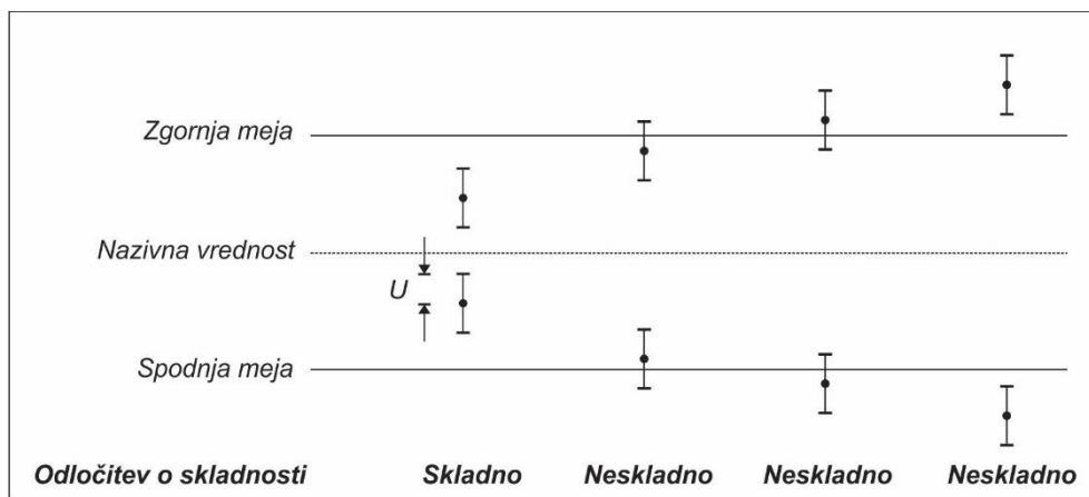
Slika 49: Pravilo odločanja z upoštevanjem merilne negotovosti meritve
