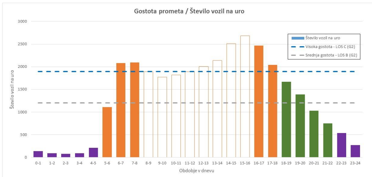
Slika 6: Tipični primer porazdelitve števila vozil v dnevu
