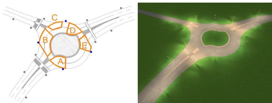
Slika 36: Primer postavitve svetilk za osvetlitev turbo krožnega križišča
