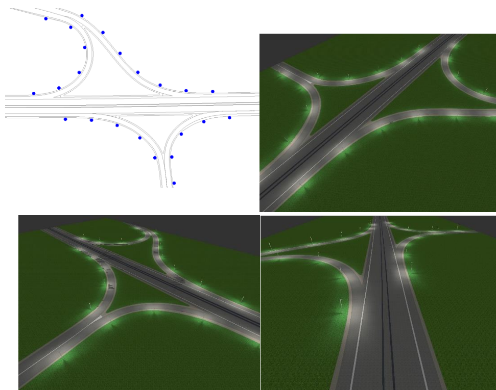
Slika 21: Primer postavitve svetilk za osvetlitev uvoza in izvoza na avtocesto oziroma hitro cesto
