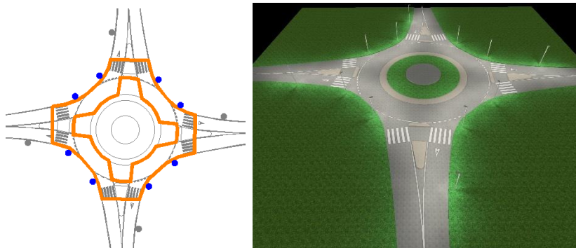
Slika 35: Primer postavitve svetilk za osvetlitev krožnega križišča z vključenimi prehodi za pešce
