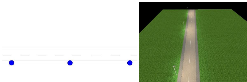
Slika 13: Primer postavitve svetilk na eni strani ceste za osvetlitev površin za pešce na neobremenjenem delu ceste v naselju
