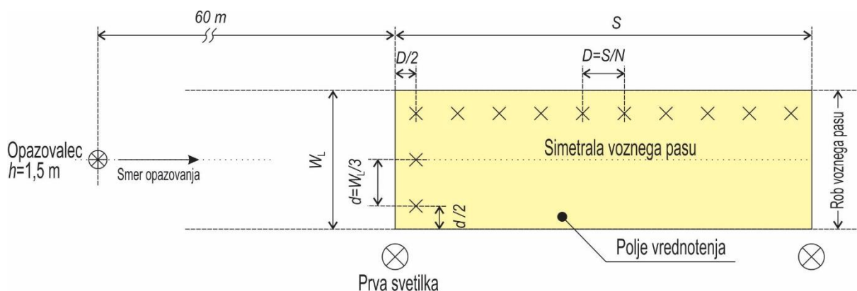
Slika 44: Postavitev merilnih točk na posameznem voznem pasu za meritev svetlosti
