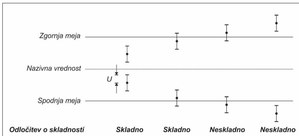
Slika 48: Pravilo odločanja brez upoštevanja merilne negotovosti meritve
