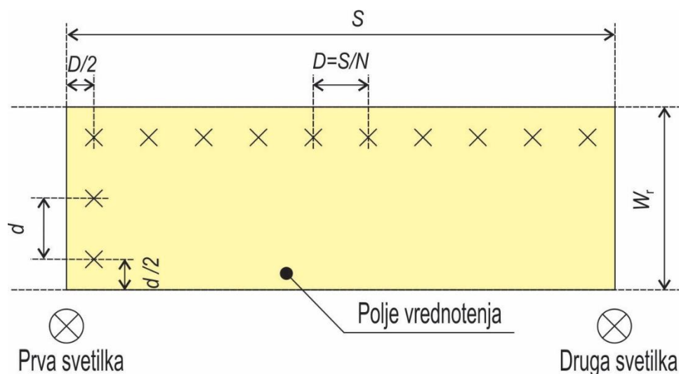
Slika 45: Merilna mreža pri meritvi osvetljenosti
