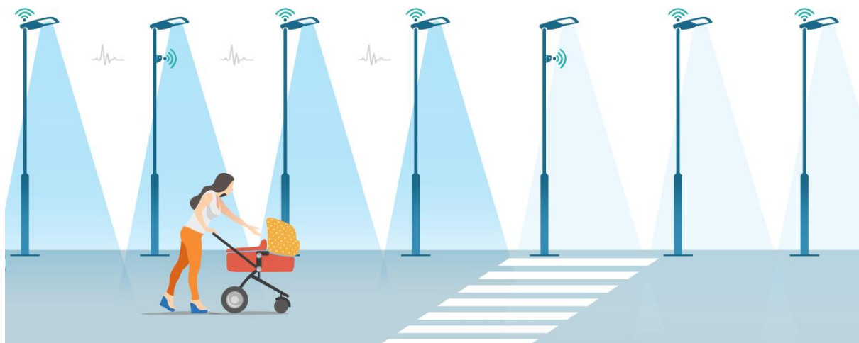
Slika 50: Prikaz delovanja pametne (dinamične) razsvetljave, kjer se ustrezne razmere zagotavljajo glede na prisotnost udeležencev v prometu s pomočjo senzorjev in komunikacije med svetilkami in nadzorno postajo
